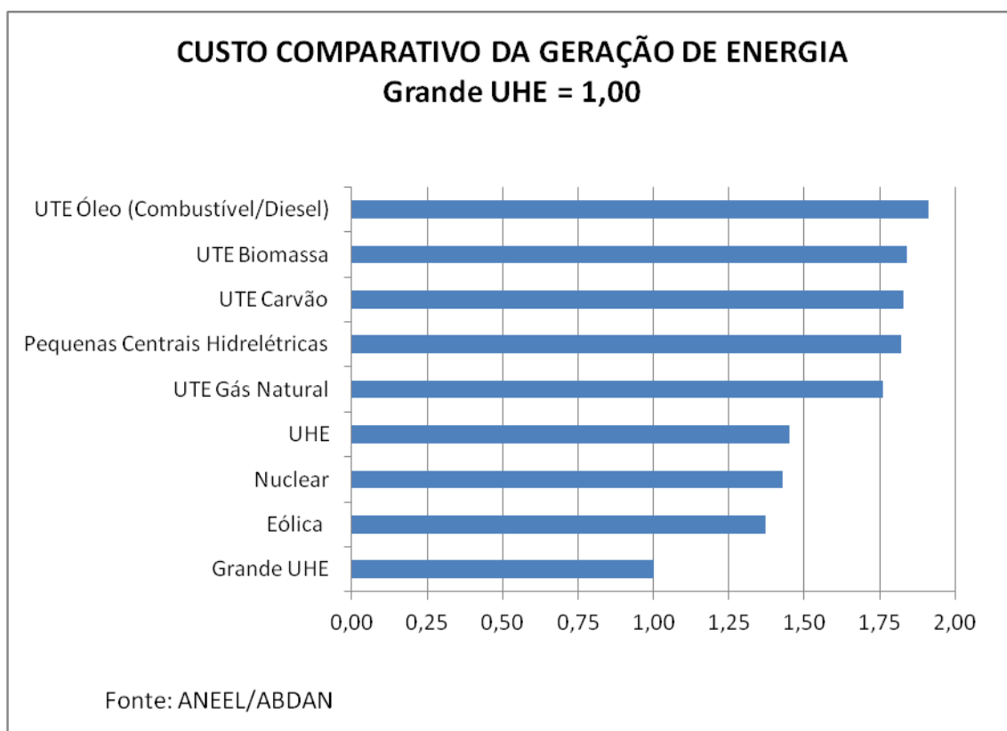
Figura 37: Custo relativo dos diversos processos para a produção de energia elétrica
